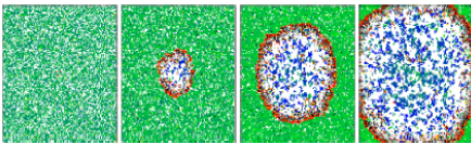
Ausbreitung einer Krankheit als Prozess in einem Teilchensystem
