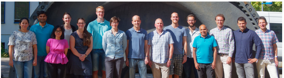
AG Technomathematik
