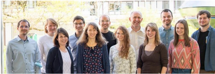
AG Statistik
