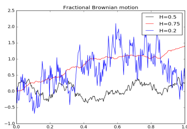
Fraktionale Brown'sche Bewegung für verschiedene Hurst-Parameter H \in \{0,5; 0,75; 0,2\}
