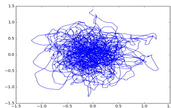
Langevin-Fadenniederlegungsmodell
