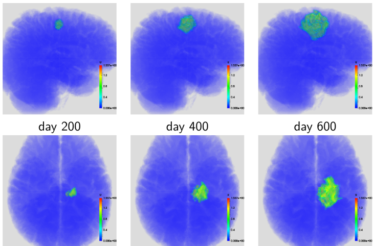
Ausbreitung eines Gehirntumors
