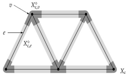
Ein netzwerkartiges Gebiet 2
